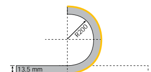
Biegeradius (Leuchtfäche aussen) bending radius (outer lighting area) rayon de courbure (surface d'éclairage extérieure)
